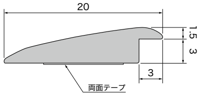
断面図 (単位: mm)
