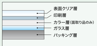
断面図
